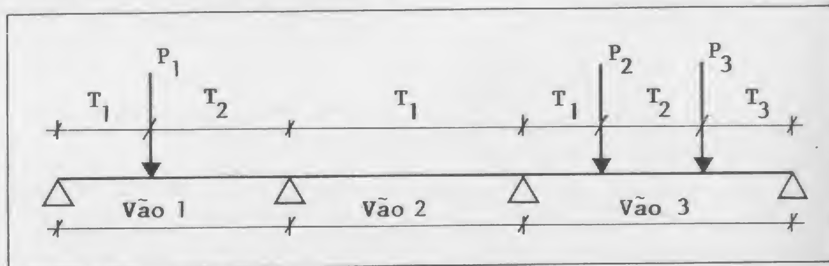
Figura 1 - Trechos de uma viga contínua
